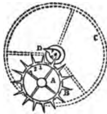
Duplex Escapement.
