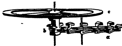
Horizontal Escapement.
